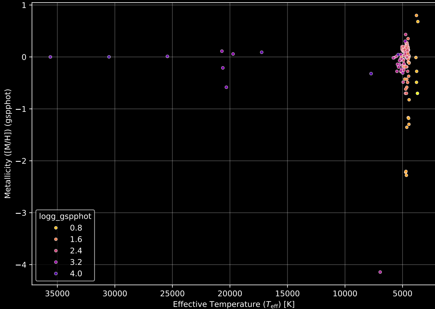
APOGEE DR17 Field: [Per_W] Stellar Population Parameters (n= 152)
